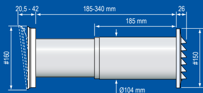
TL 100DE 經典型
