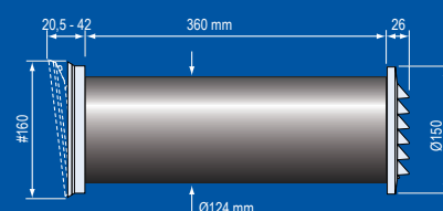
TL 80DE-dBs 降噪型
