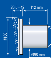
TL 100DE 經典內風罩
